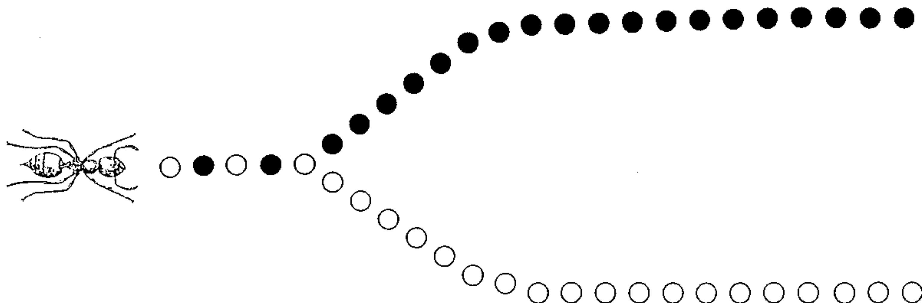
Fig. 2: La piste à bifurcation. La base est composée d'un mélange de la moitié de la concentration de chaque branche.
